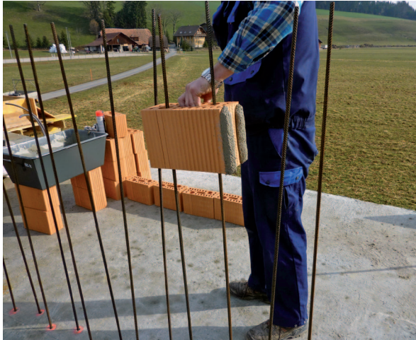
4. Einfädeln des Steines mit aufgebrachtem Stossfugenmörtel (Spatz).
